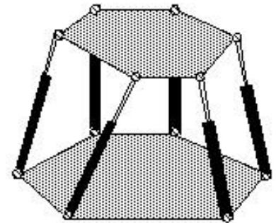
Plate-forme de Stewart: plusieurs chaînes fermées
