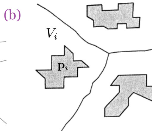
Graphe de Voronoï : Générateurs de dim. 2 (surfaces)
