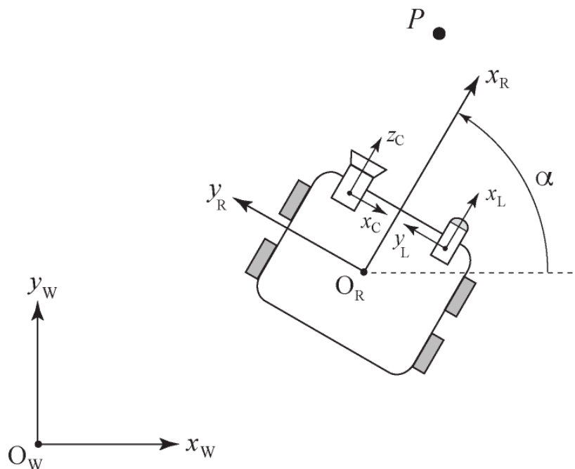
Figure 2: Robot mobile avec caméra et laser embarqués.
