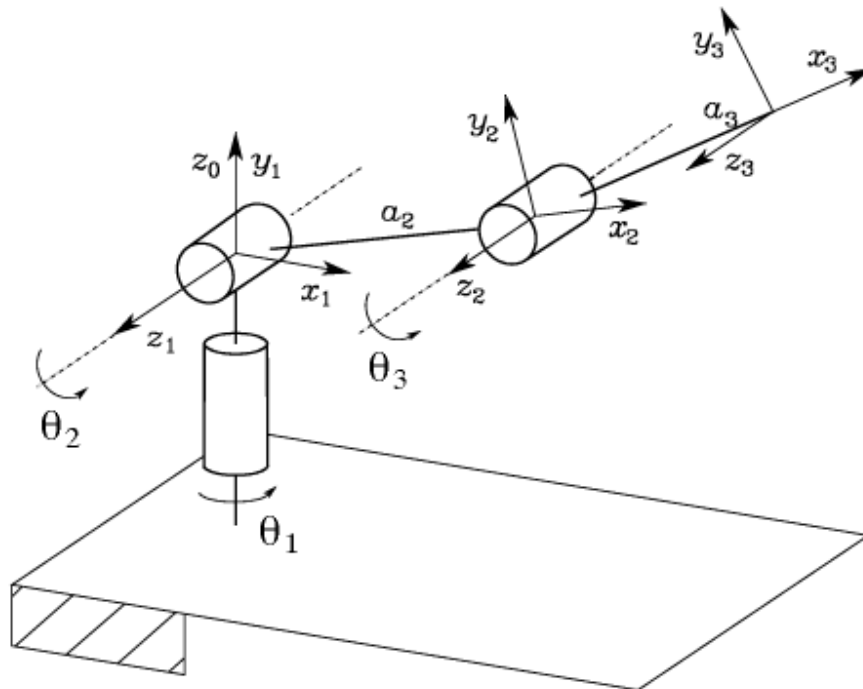
Figure 1 : Manipulateur anthropomorphe.
