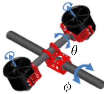
Rotors duaux: 1 des 4 modules du drone
