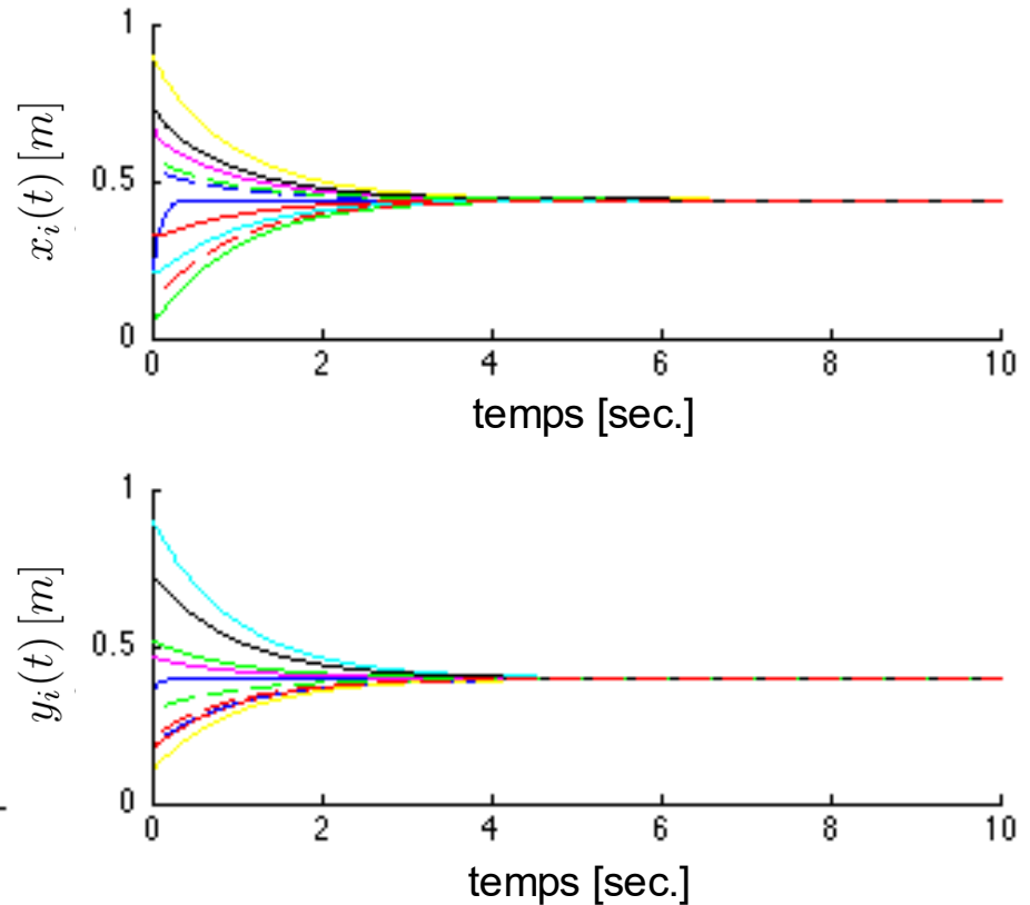
Évolution temporelle des coordonnées x et y des 10 robots
