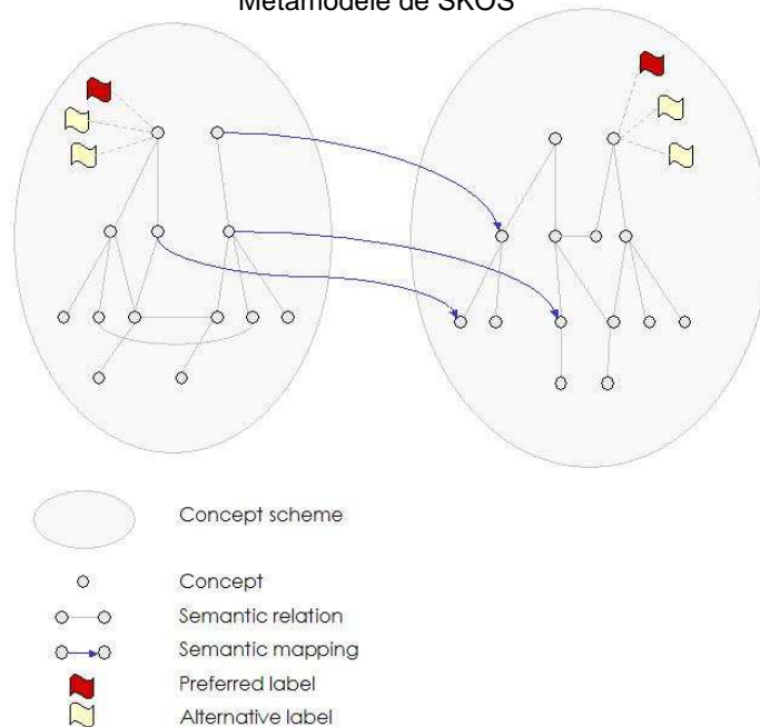
Métamodèle de SKOS
